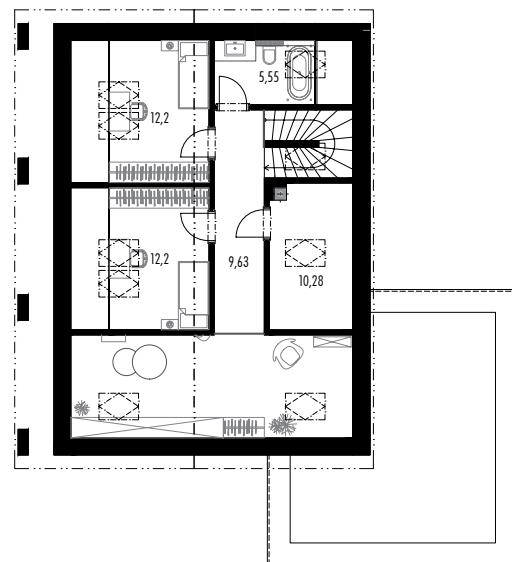
poschodie: 71,36 m 2
