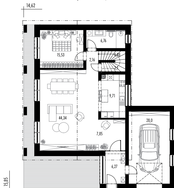
prízemie: 128,64 m 2
